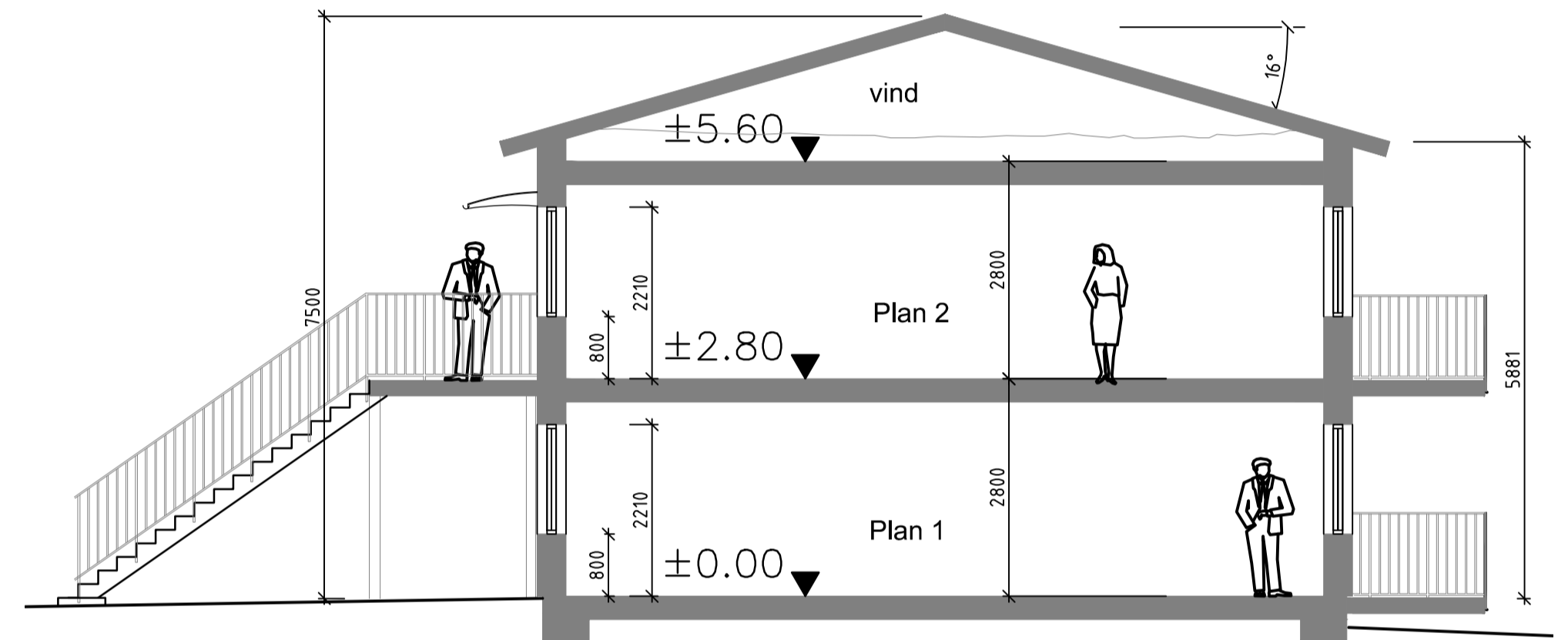
SEKTION
